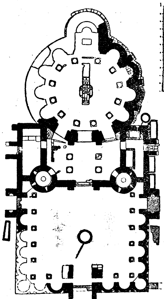
Планъ на „Златната църква“ въ манастира при „устието на Тича“. Планъ на архит. Ал. Рашеновъ.
