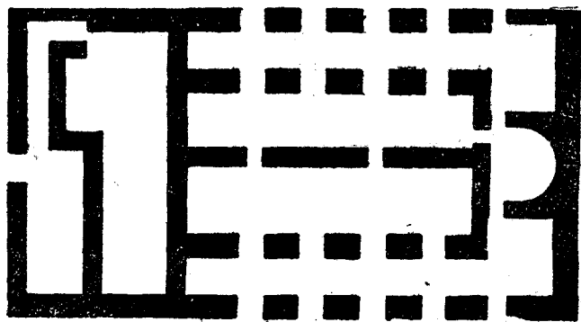
Тронната палата въ Плиска. Планъ на К. Шкорпилъ.
