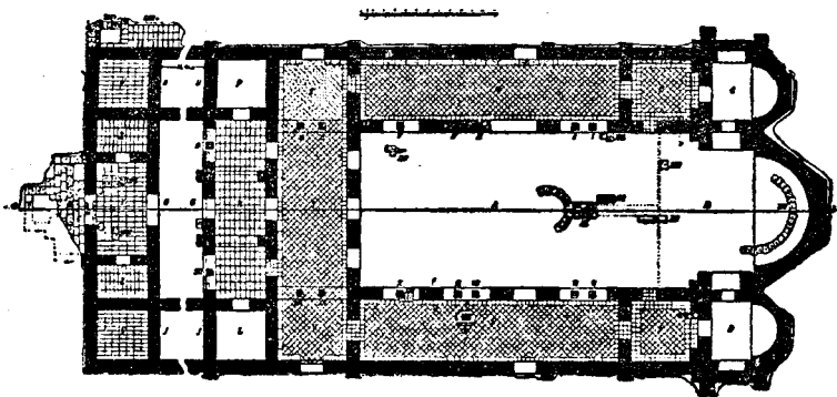
Планъ на голѣмата църква въ Плиска. По К. Шкорпилъ.
